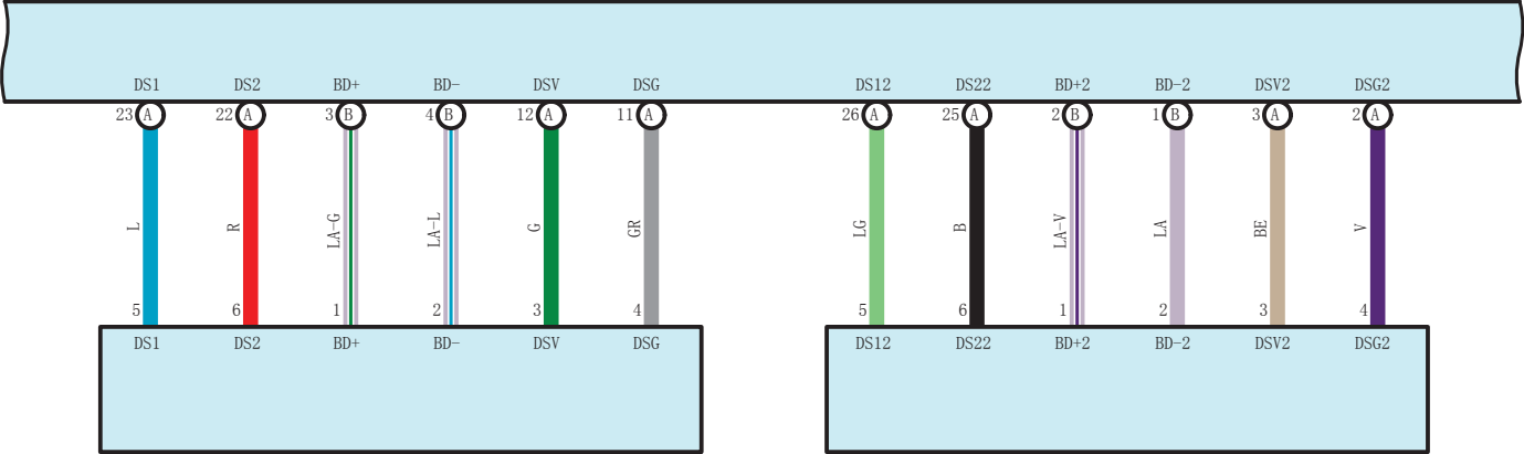
Y19 左侧电动背门单元总成组件
